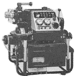
可搬消防ポンプ (ボールロック放水バルブ仕様)
